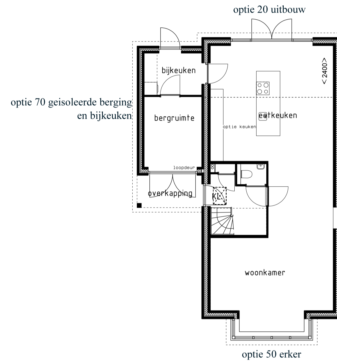
Begane grond
