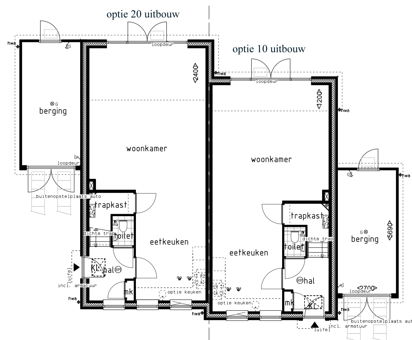
Begane grond
