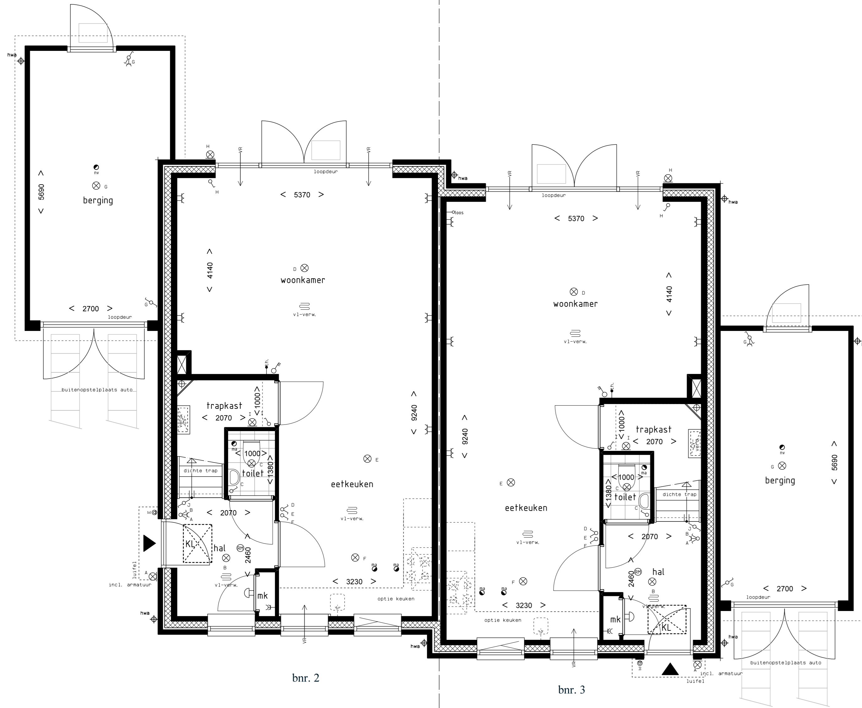
Begane grond
