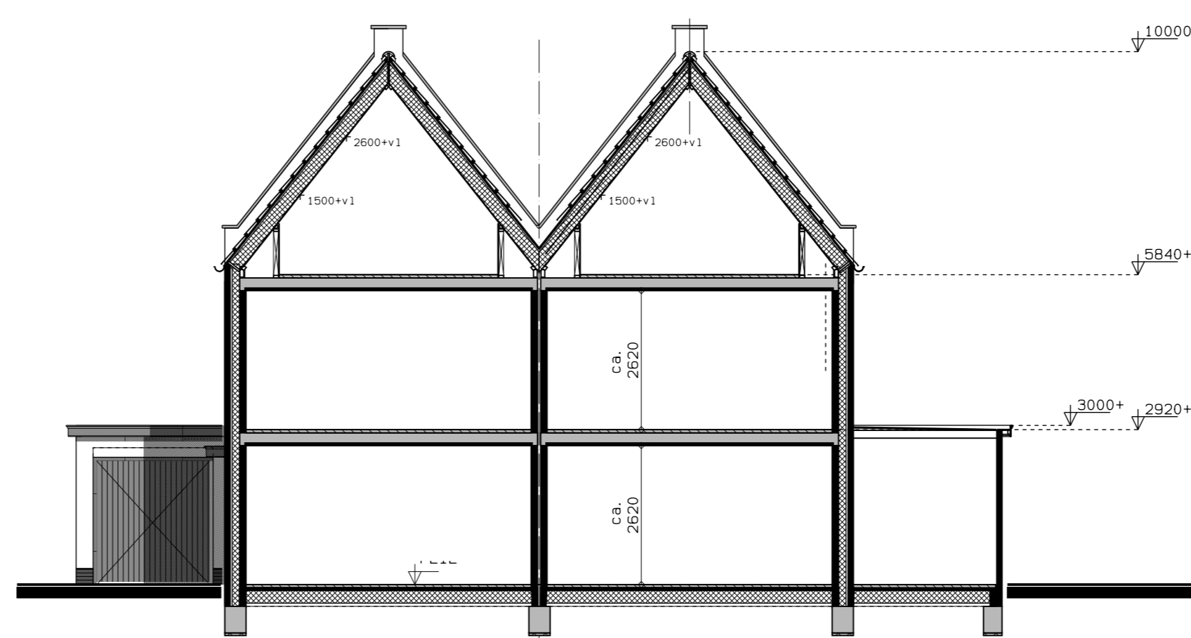
Doorsnede A-A
